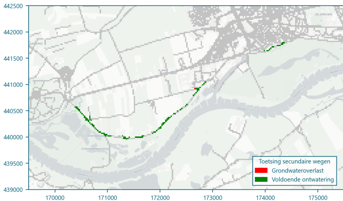
Afbeelding 4.15 Toetsing ontwatering van secundaire wegen met een ontwateringsdiepte van 0,7 m bij de Gemiddeld Hoogste Grondwaterstand (GHG) van 2009-2017 van ontwerploop 2
