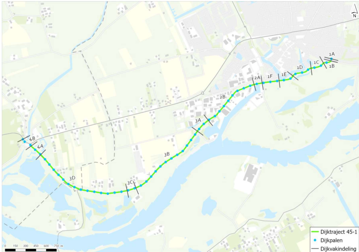
Afbeelding 1.1 Dijkvakindeling Grebbedijk. 1=stedelijke dijk, 2=Nudedijk, 3=landelijke dijk, 4=Hoornerk
